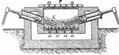
Fig. 151. — Four Crampton.
